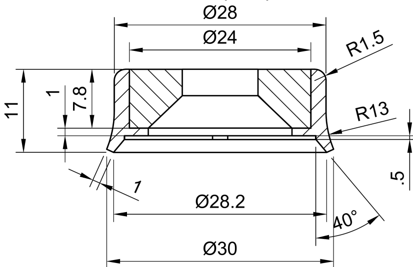
A-A (2:1)
